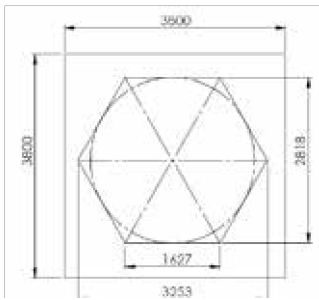
25 Ton silo concrete dimensions
